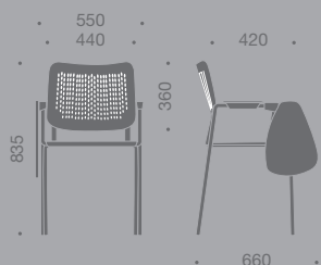
MIA1+ tablette écritoire + writing table + atril escritorio
